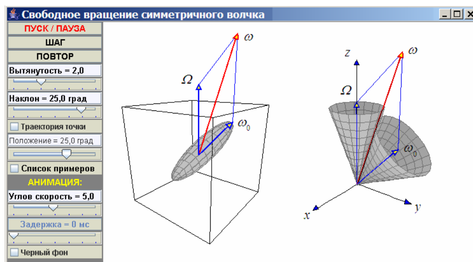
Рис. 3. Окно моделирующей программы с иллюстрацией свободного вращения симметричного волчка вытянутой формы (слева) и геометрической интерпретацией этого вращения (справа).
