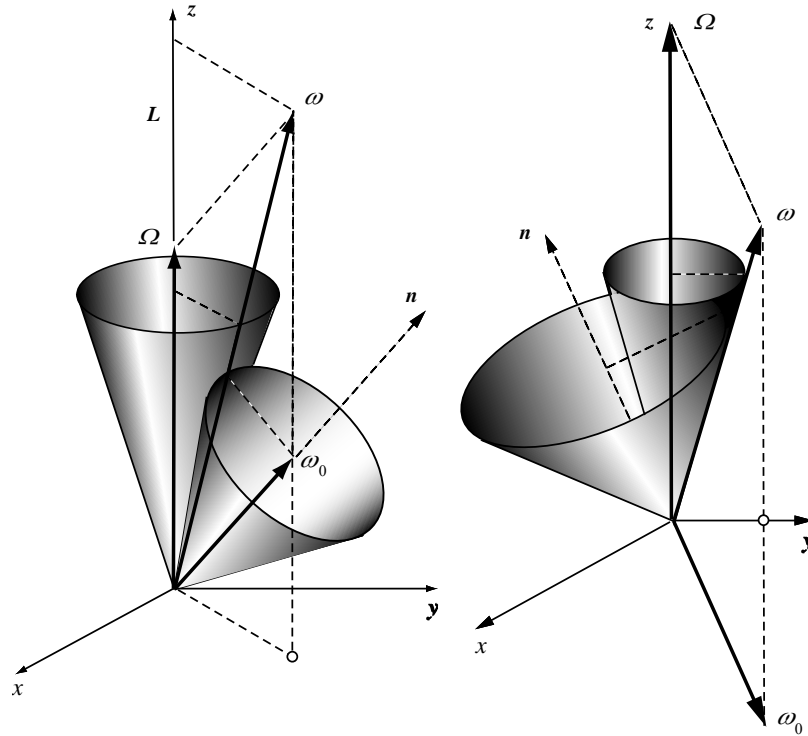
Рис. 2. Геометрическая интерпретация свободной прецессии симметричного волчка как качения без проскальзывания мысленно связанного с телом подвижного аксоида по поверхности неподвижного аксоида ( \omega = \omega_0 + \Omega ).
